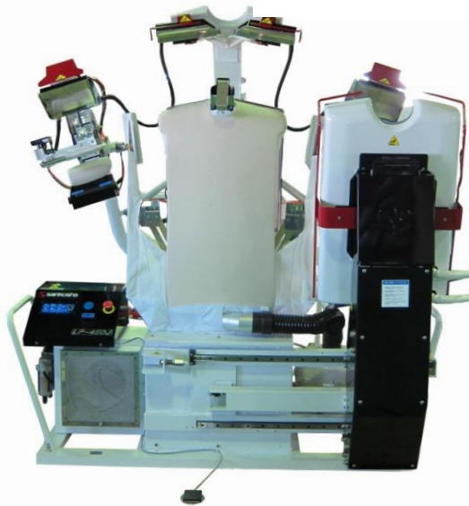
衬衫机 LP-450J
